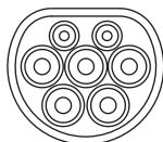
TIPO 2 (Mennekes) VDE-AR-E 2623-2-2
